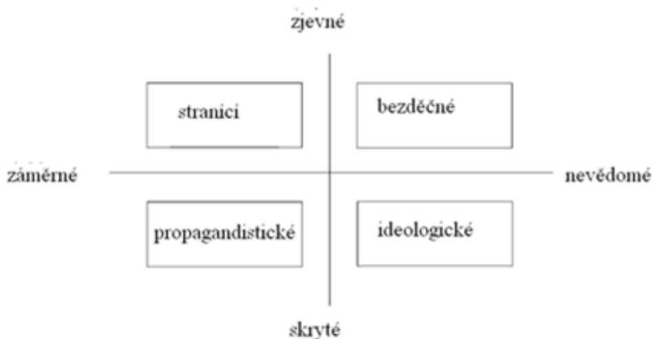
Obrázek 2: Typologie předpojatosti
